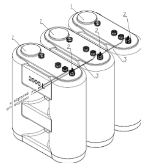
Рис.4 Двухтрубная система
